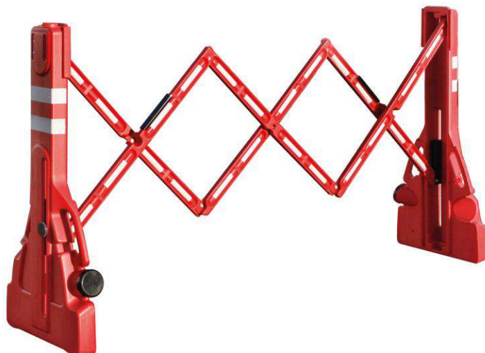
Bariera nożycowa ze zintegrowanym systemem składania materiał wykonania: PVC wysokość: 1100 mm; szerokość: rozciąganie do 2200 mm. Ustawienie: oba końce bariery mogą być wypełnione piaskiem lub wodą w celu zwiększenia stabilności. cena - 294 zł
