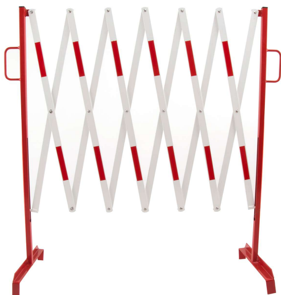
Barierka nożycowa długość max 3 mb materiał wykonania: stal ocynkowana zabezpieczenie antykorozyjne (malowanie proszkowe) wysokość 1100 mm; waga 10 kg cena - kontakt telefoniczny
